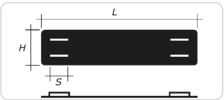
Hållare för enteckenmärke eller färdigskrivet flerteckenmärke.
